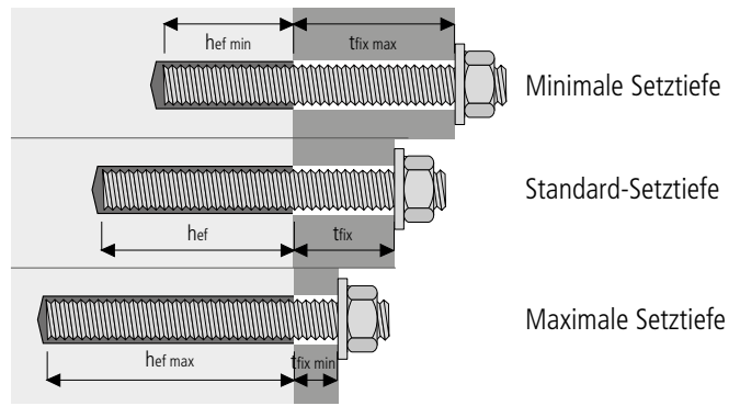
hef + tfix = Nutzbare Länge der Gewindestange (ohne Mutter und U-Scheibe)
