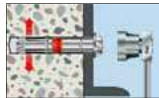
4. Vorgeschriebenes Drehmoment mit Drehmomentschlüssel aufbringen
