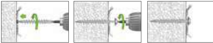
Empfohlene Spenglerschraube 4,5 x 25 mm
