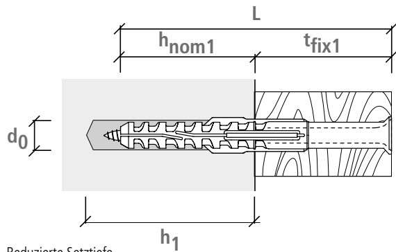
Reduzierte Setztiefe
