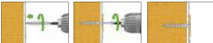
Verwendbar mit Schrauben \varnothing 4,0\text{ mm} ; Schraubenlänge 15-20 mm + Anbauteildicke
