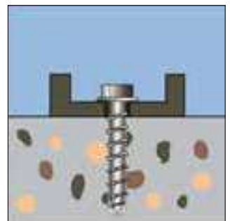
4. Fertig
