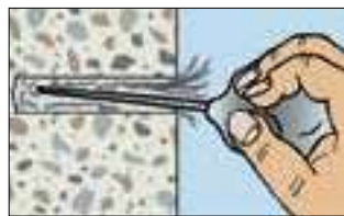
2. Bohrloch reinigen
