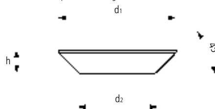
Geometrie Senkkopf bei Ausführung SZ-SK.
