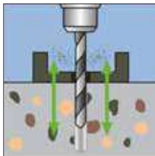
2. Bohrloch reinigen
