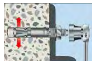
4. Vorgeschriebenes Drehmoment mit Drehmomentschlüssel aufbringen.
