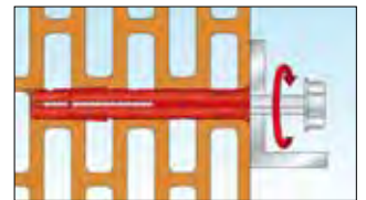
4 Schraube anziehen
