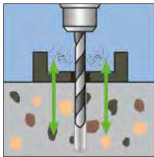
2. Bohrloch reinigen
