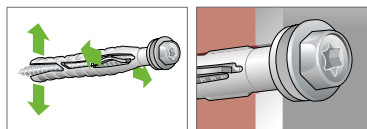
MFR FB SSKS Flachbunddübel mit Sechskantschraube mit angepresster Scheibe Stahl verzinkt / Edelstahl A4 Art.-Nr. 0905 98. ...
