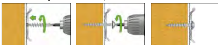
Empfohlene Spenglerschraube 4,5 x 25 mm
