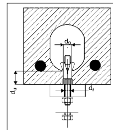
RECA Hohldeckenanker Easy im gespreizten Zustand.
