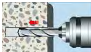
1. Loch bohren.
