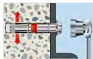
4. Vorgeschriebenes Drehmoment mit Drehmomentschlüssel aufbringen
